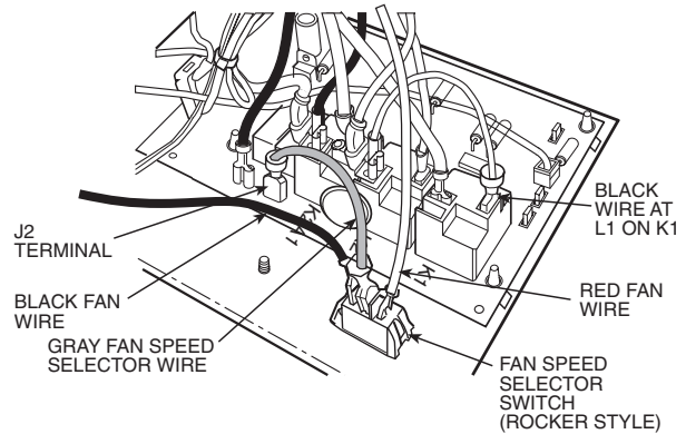
Fig. 4 — Fan Speed Selector Wire
