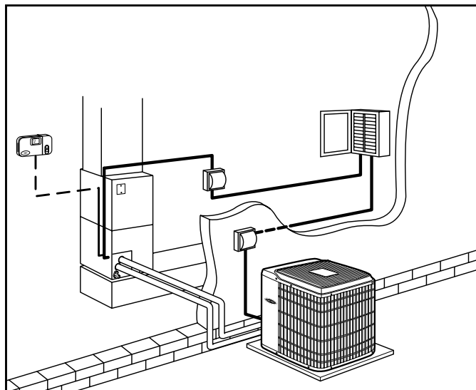
Fig.1—Instalación típica del sistema doble.
