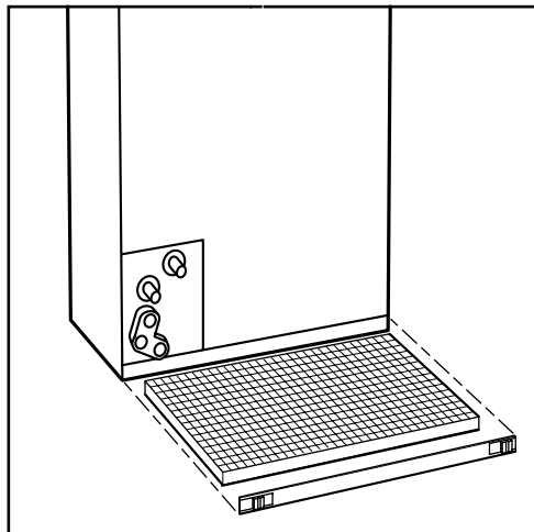
Fig. 5—Extracción del filtro del serpentín ventilador
