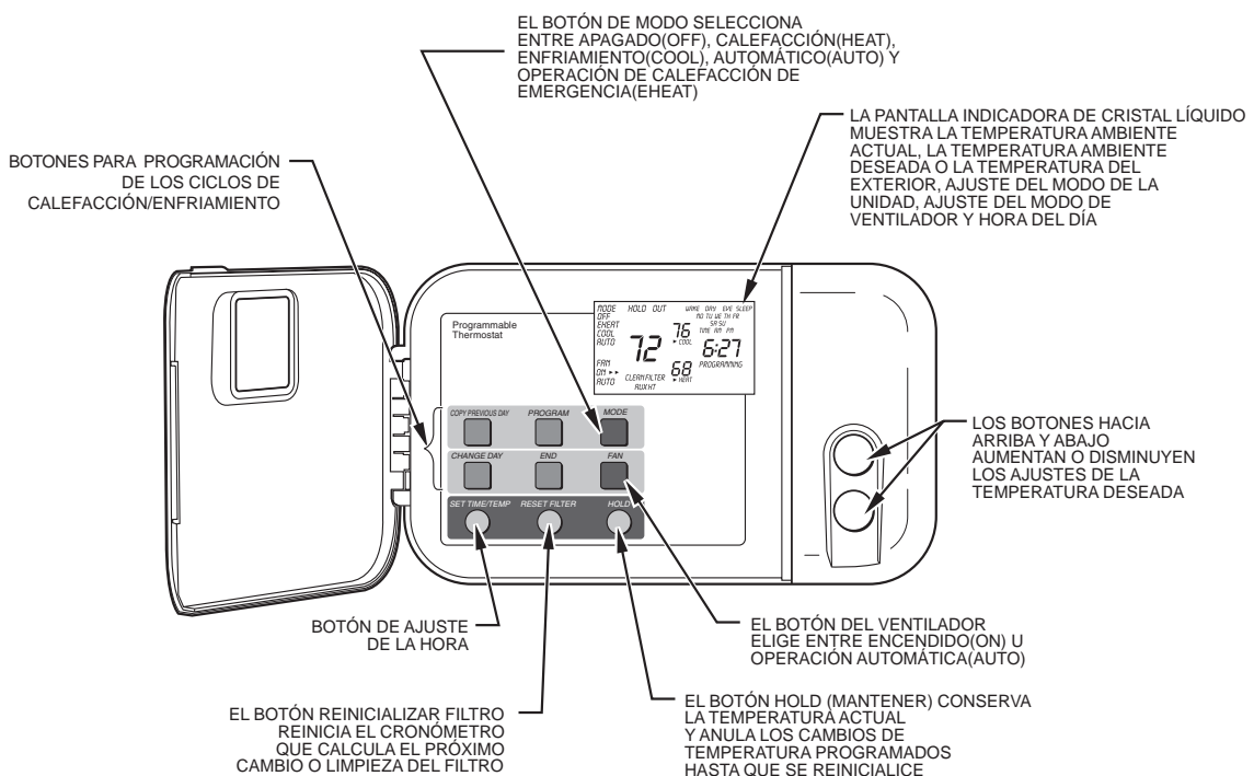
Fig. 3—Termostato típico programable Carrier
